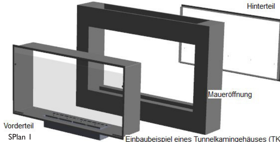
Einbaubeispiel eines Tunnelkamingehäuses (TKG)
